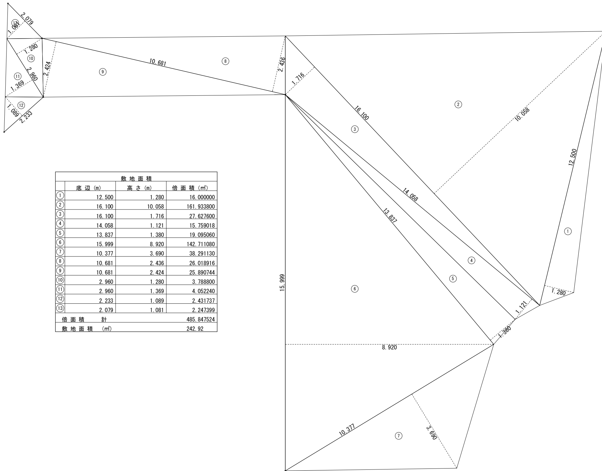
敷地測量図 S:1/100
